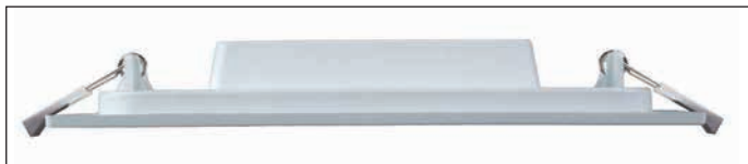
Upevňovací držák s pružinami pro vestavnou montáž do sádkartonového stropu
