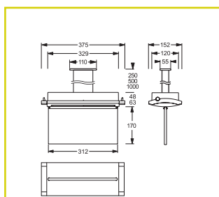
Trubkový závěs
