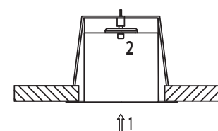
Obr. 13) ROZEPŘENÍ PRUŽIN
