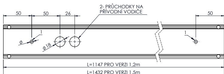
Obr. 4) MONTÁŽNÍ OTVORY
