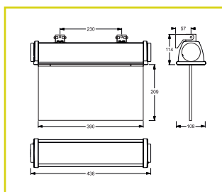
Nástěnná a stropní montáž na nastavitelnou konzolu
