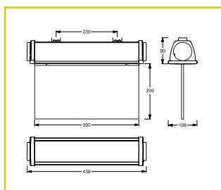
Přisazená nástěnná a stropní montáž
