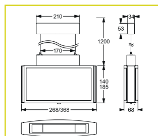
Seilpendel
