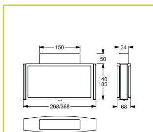
Deckenanbau
