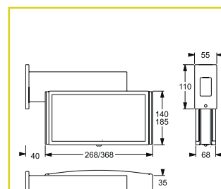
Ausleger
