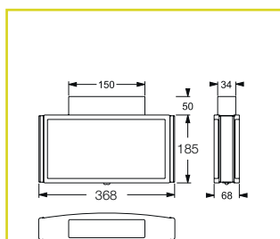
Deckenanbau
