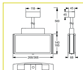
Rohrpendel
