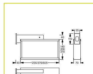
Ausleger
