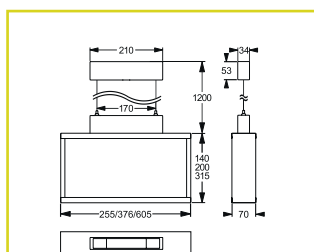
Seilpendel
