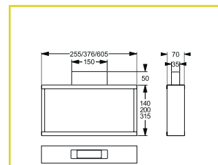
Deckenanbau
