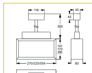
Rohrpendel rund
