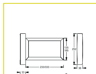
Ausleger
