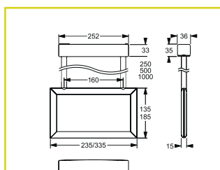
Rohrpendel
