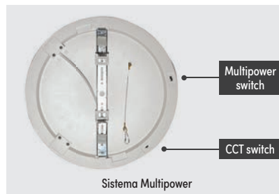
Staffa removibile dotata di posizioni preimpostate per adattarsi a diametri di fori differenti: 12W fori compresi fra 55 e 200mm 18W fori compresi fra 55 e 280mm
