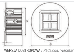
WERSJA DOSTROPOWA / RECESSED VERSION
